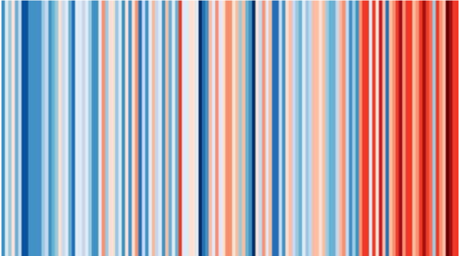
Strichcode der Durchschnittstemperatur für Deutschland zwischen 1881 und 2017; jeder Streifen steht für ein Jahr. Grafik: Ed Hawkins/klimafakten.de
